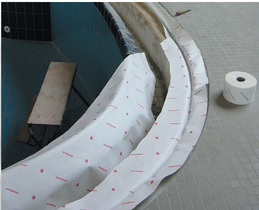
Szkody wynikające z nieszczelnej szczeliny dylatacyjnej
