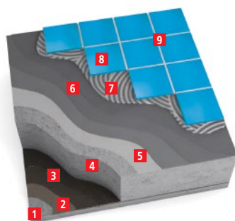
Rys. 3 Schemat systemu dla dna niecki basenu.
