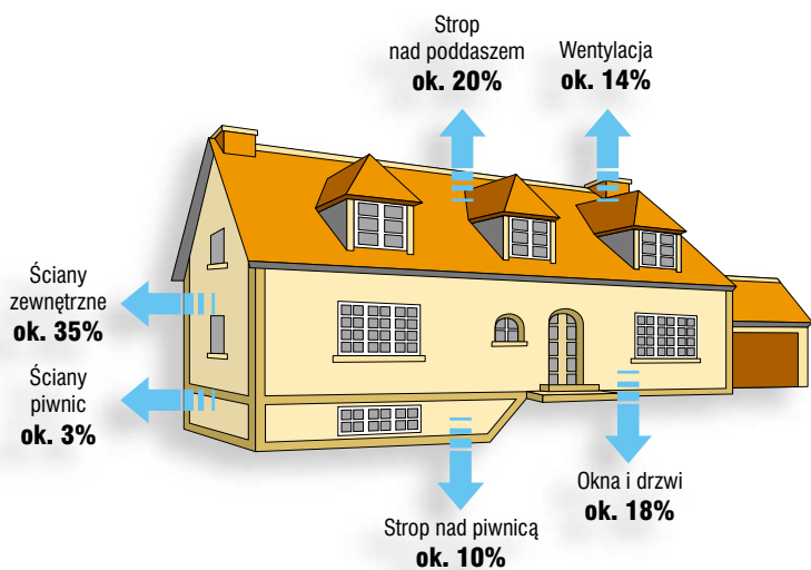
Rozkład strat ciepła w budynku jednorodzinny
